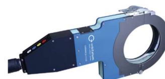
ORBIWELD 115S
